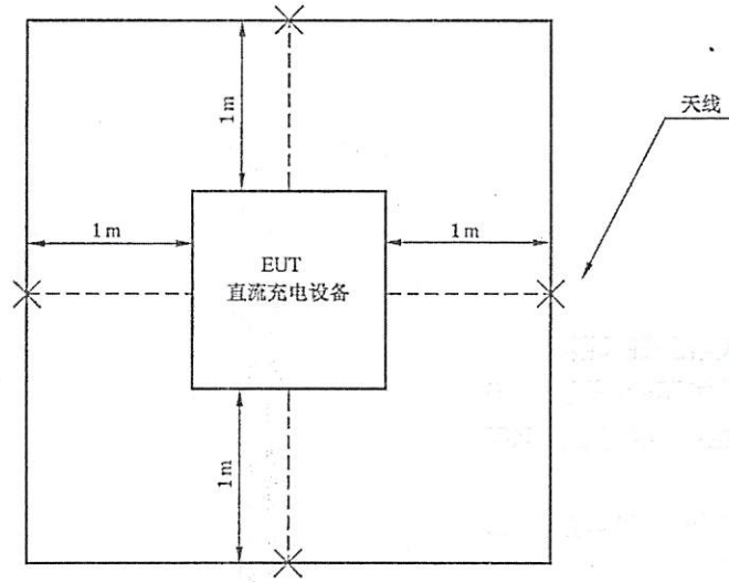
a) 俯视图
