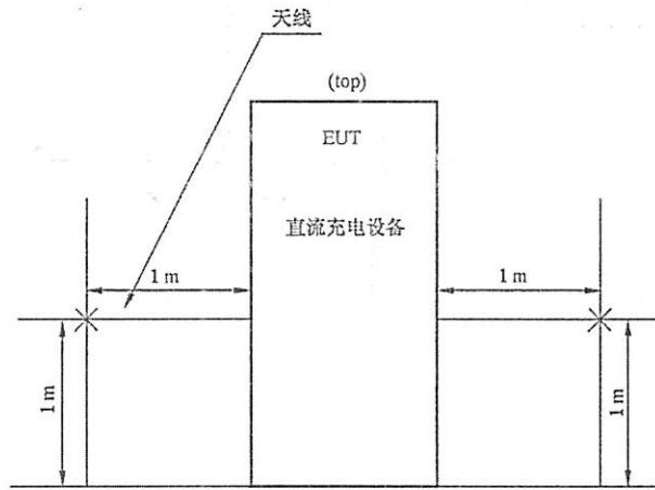
b) 侧面图
