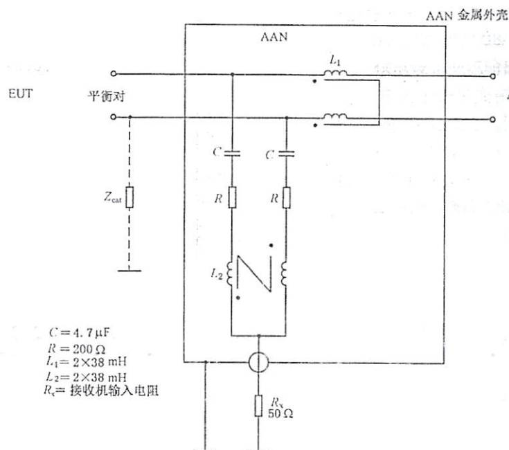
图 B.1 ISN 对称通信线的示例
