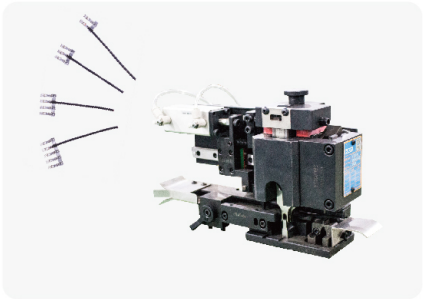
AFTCA 计数切断型压接模具
