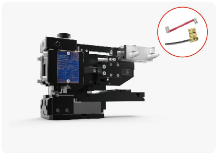
NEFTCA-X 型旗形端子压接模具
