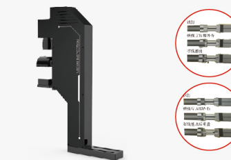
CVS-A30 端子检测系统
