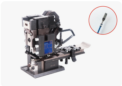
E4 型压接模具
