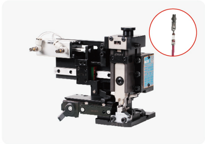
YJM-AFS300I 型压接模具
