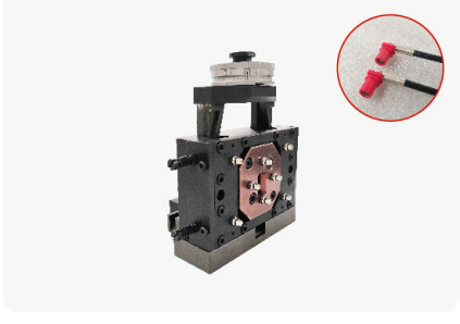
RFPCA 压接模具
