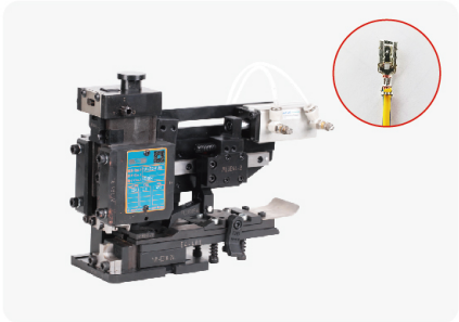
YJM-AFE300I 型压接模具
