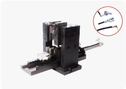
CLM 轻型电瓶端子压接模具
