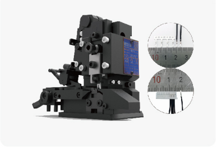
Nano 型压接模具 (S4B)
