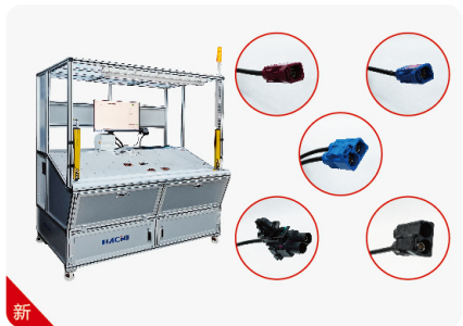
HCS-F FAKRA线束通检测台
