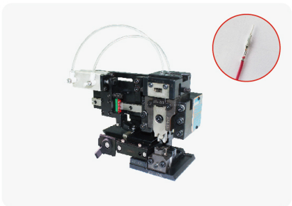
AS4A 型压接模具
