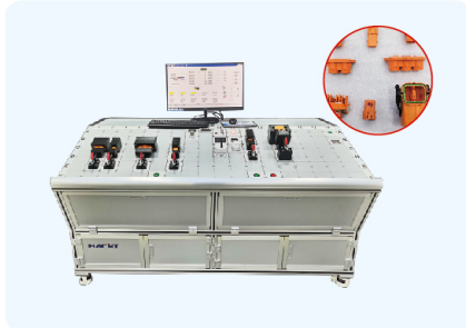
GZ-0012 气密导通检测台
