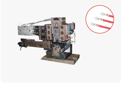
LCMS 型重载压接模具
