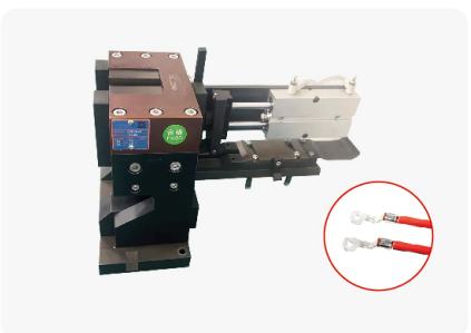
LCME 型压接模具
