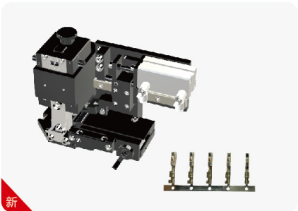
ADS 右进料压接模具
