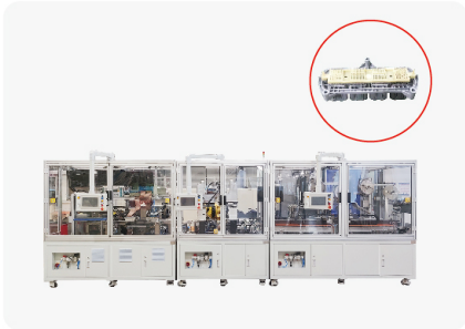
HBQ-K612 168W板端连接器设备
