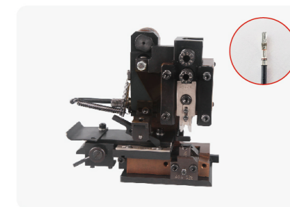
YJM-4XA 模具
