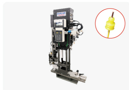
FSA-001E 型防水栓工作站
