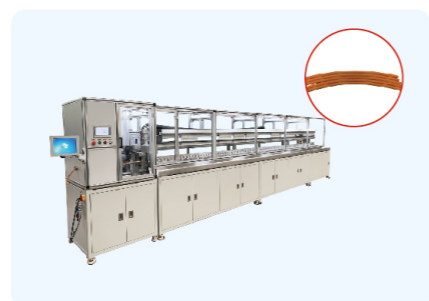
HBQ-433 高精度拉线裁线机
