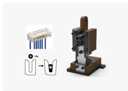
DYM-C 刺破压接模具
