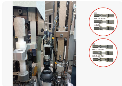
CVS-A30 端子检测系统
